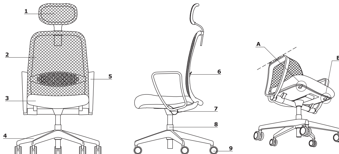
A - regulacja wysokości siedziska, B - blokada oparcia
