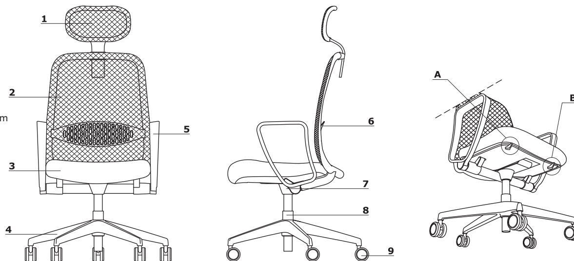
A - réglage en hauteur du siège, B - blocage du dossier
